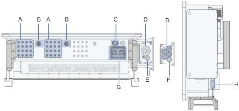
Figura 5-2 Descrição do terminal (SG75CX-P2)
