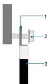
Figura 5-4 Conexão do cabo de alumínio
